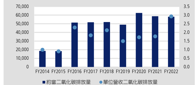
圖 33：碳排量
